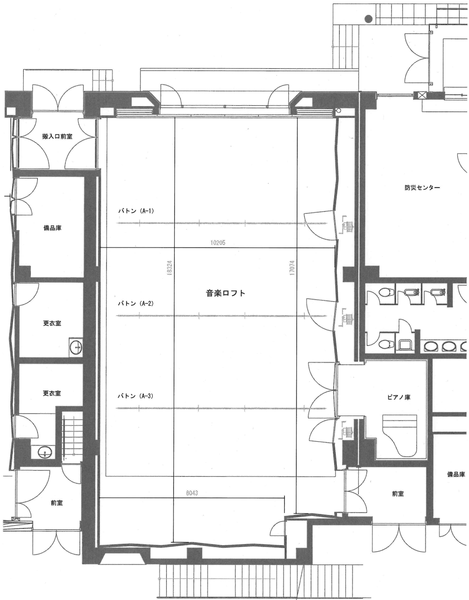
可児市文化創造センター 音楽ロフト 平面図 1/100
